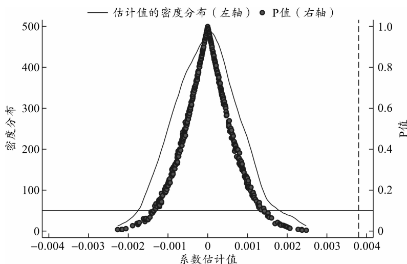
图3 安慰剂检验
